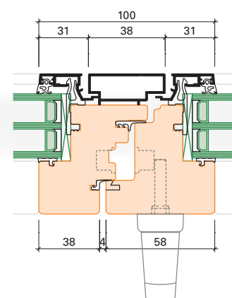
Mittelpartie (Massstab 1:3)
