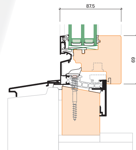
Vertikalschnitt (Massstab 1:3)
